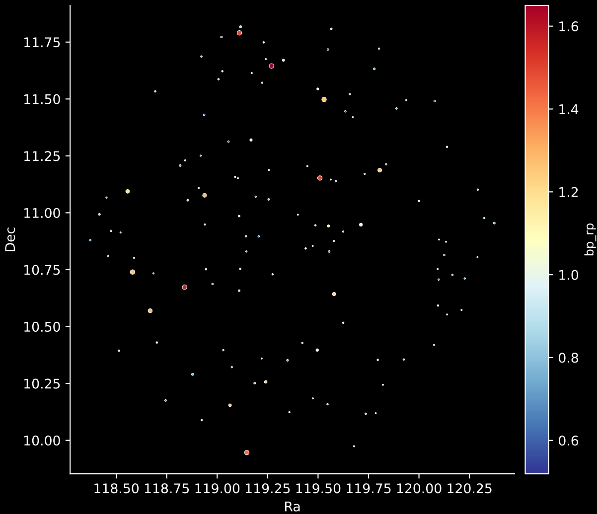
GALAH DR4 Field: [6680] Stars: 120
