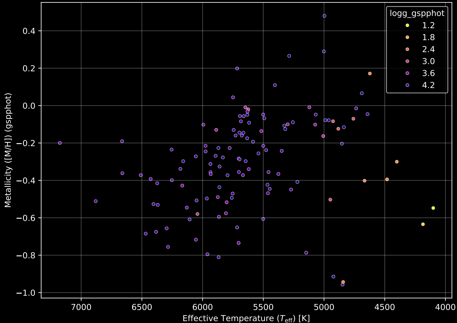
GALAH DR4 Field: [6680] Stellar Population Parameters (n= 120)
